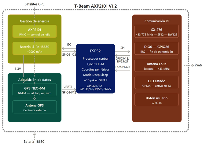
Figura 5: Diagrama de bloques funcionales del sistema.
