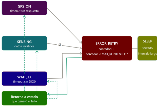
Figura 10: Ruta de manejo de errores del sistema.
